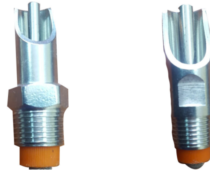
Bebedero de 3/8 con rosca de 1/2
